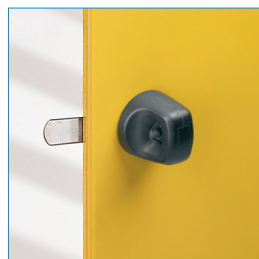
Sicherheits-Drehriegel als „Freidreher“, wird lose mitgeliefert, leichte Selbstmontage
