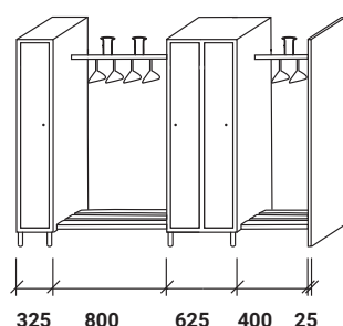
Serie 130 Aufstellungsbeispiel
