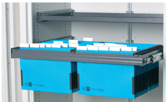
Ausziehbare Hängeraahmen mit Sonderausstattung: Sicherheitsauszugsverriegelung / Einzelverriegelung je Auszug (Sonderausstattung)
